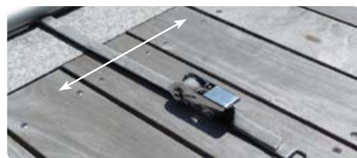
Edelstahlratsche mit Gurt und Ring (seitlich und in der Tiefe verstellbar)
